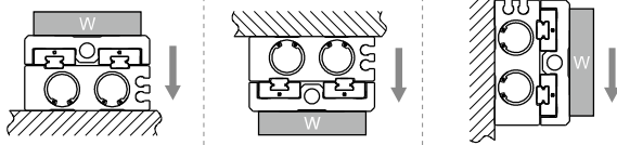
Fig. 1 : Applied load
